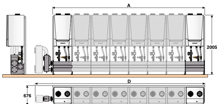
Kessel in Reihe auf Gerüst Bodenstehend „LV“
