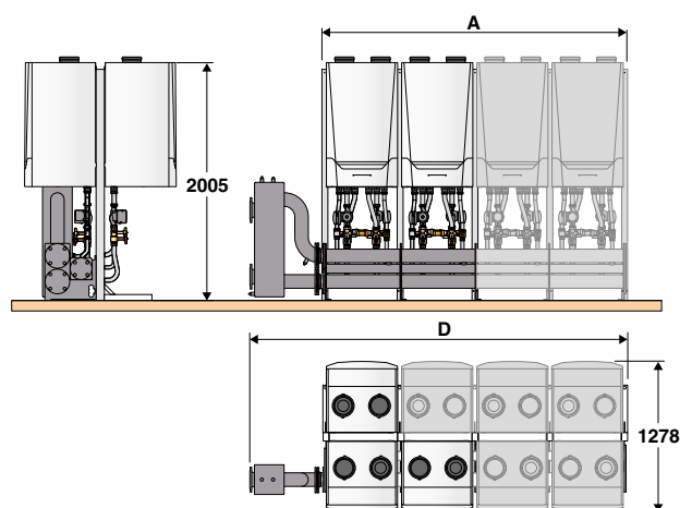
Kessel Rücken an Rücken auf Gerüst „RG“
