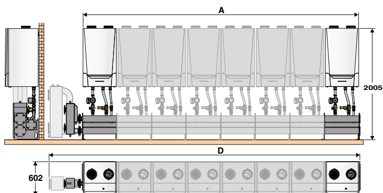
Kessel in Reihe an der Wand „LW“
