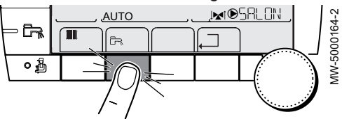
Abb.22 Aufrufen des Modus Warmwasserbereitung
