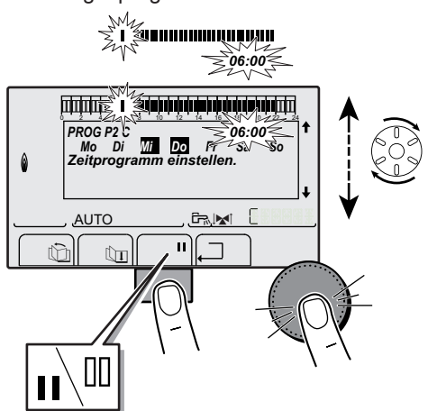
Abb.30 Auswählen/Abwählen des Tagesprogramm-Zeitbereichs
